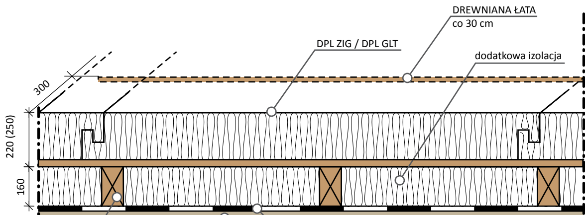
Rys. B Przekrój poziomy przez połac dachową z dodatkową izolacją międzykrokwkową.
